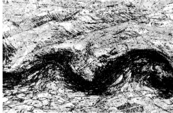
Verbindungszone (125-fach)
