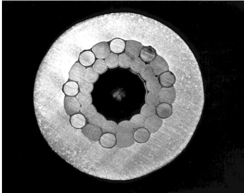
Seilquerschnitt mit Sprengschweissmuffe
